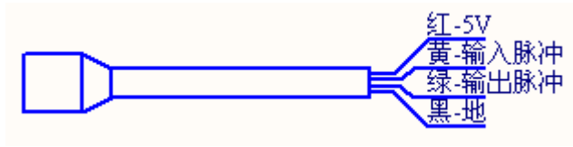
附图 1 脉冲测试线示意图
